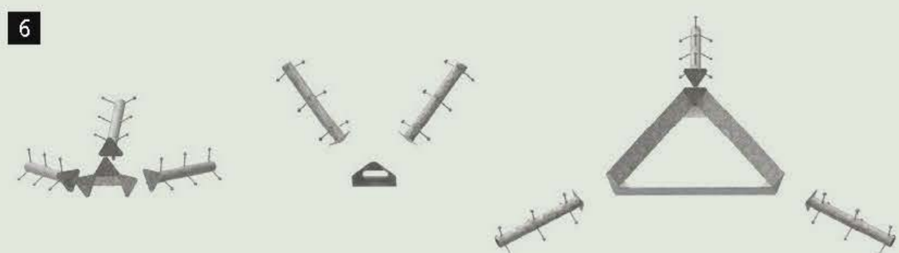
Piezas para montaje de las estructuras
